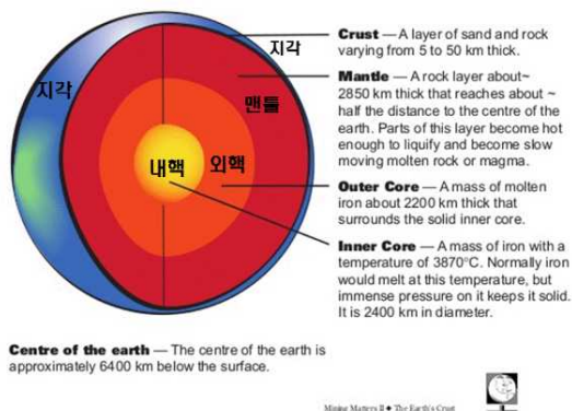
The Layers of the Earth 지구 내부구조 - 창조 첫날부터 오늘날까지 동일
